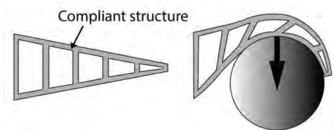
Рисунок 1. Захват типу “Fin Ray”, з виділеною м'якою структурою
