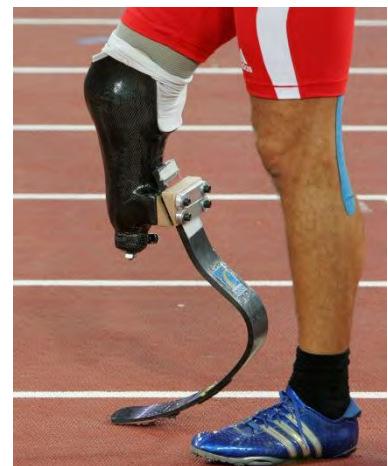
Рисунок 3. Спортивний протез
