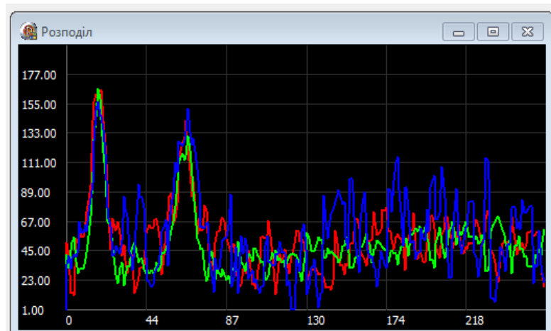
Рисунок 3. Зображення зон поверхневих дефектів кремнію в коронному козряді, які були побудовані програмою TIVC: ліворуч присутні два осередки із коронним розрядом діаметром 50 \pm 5 мкм та 70 \pm 5 мкм
