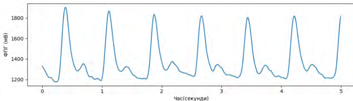
Рисунок 2. Фотоплетизмограма
