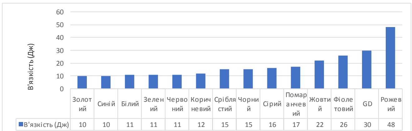
Рис. 5. Вплив кольору матеріалу на в'язкість.
