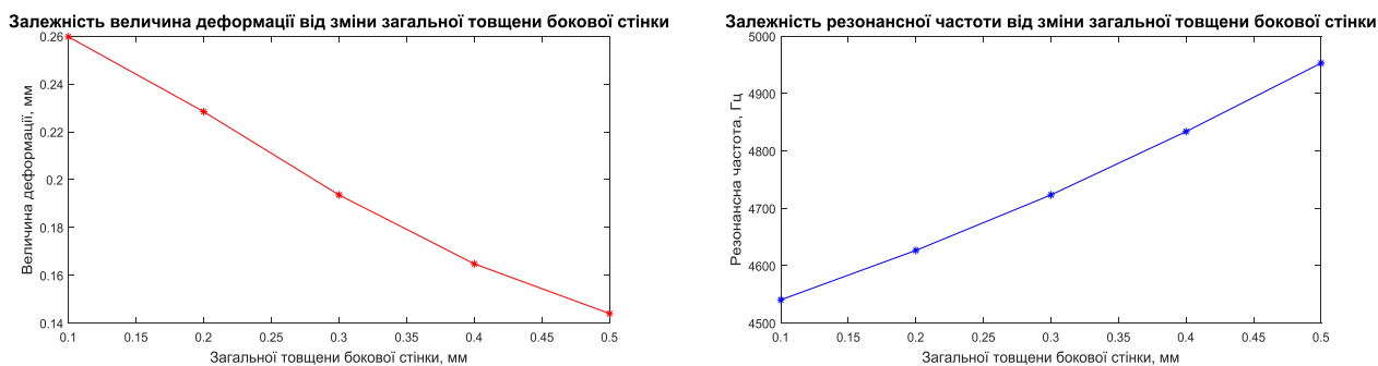
Рисунок 5. Графік залежності зміни величини деформації та резонансної частоти від загальної товщини бокової стінки
