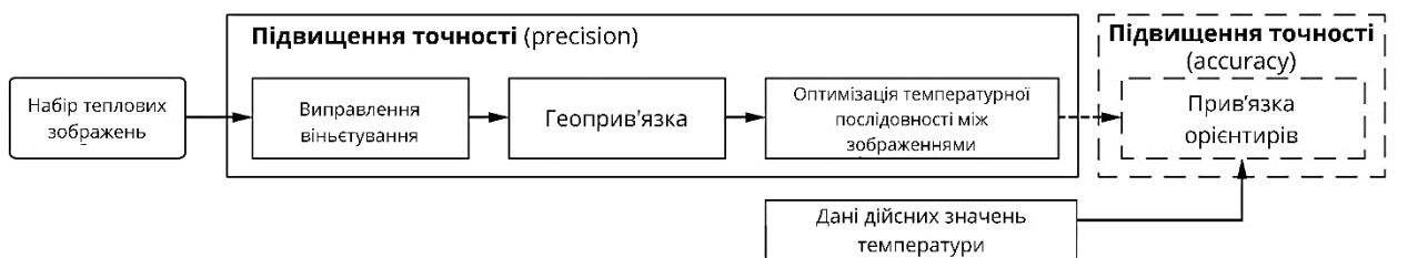
Рисунок 1. Блок-схема запропонованого методу самокалібрування, яка складається з кроків підвищення точності (суцільний прямокутник) і необов'язкового кроку підвищення точності (пунктирний прямокутник).
