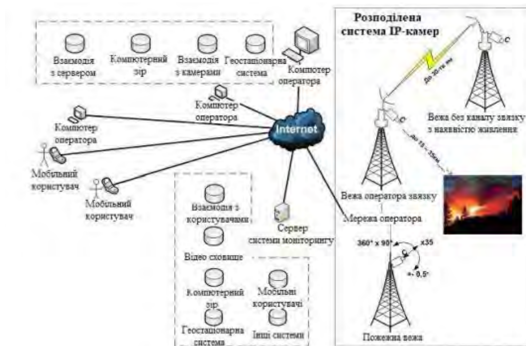
Рисунок 1.1 - Архітектура автоматизованої система моніторингу лісового господарства [2].
