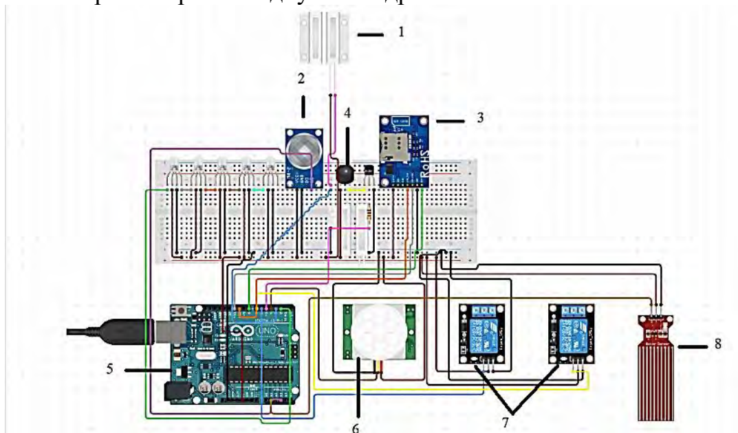
Рисунок 4. Схема підключення автоматизованого блока захисту приміщення з GSM-модулем
