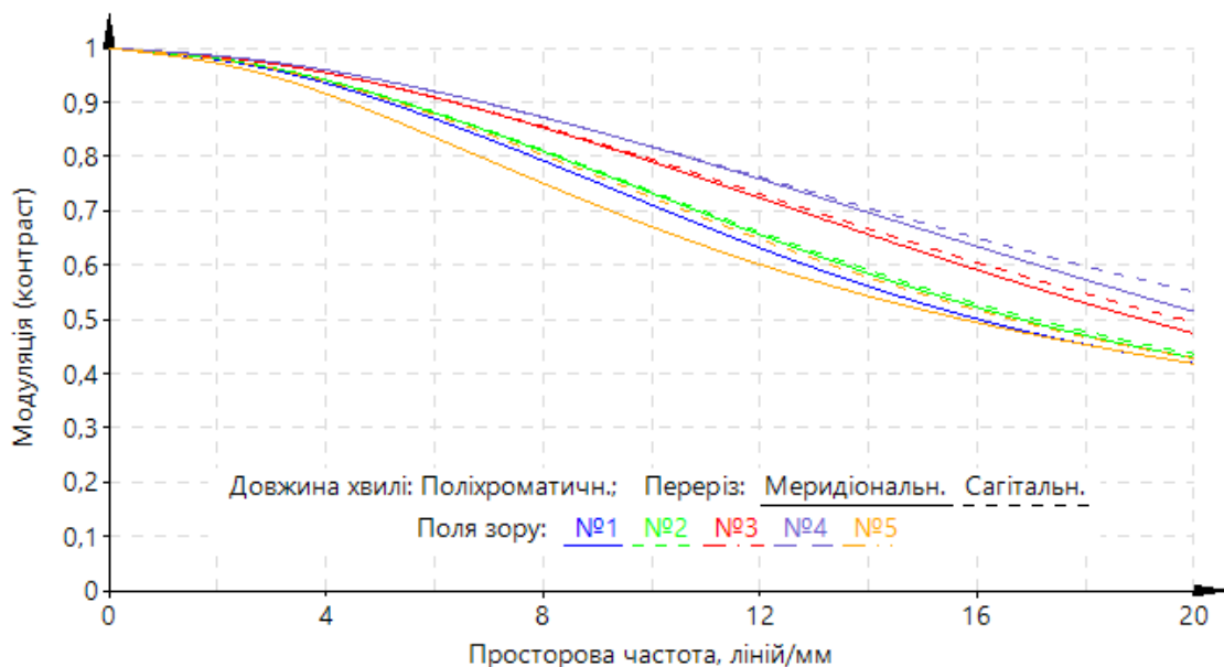
Рисунок 3. Значення поліхроматичних МПФ синтезованого об'єктива для SWIR діапазону. Поля зору №1...5 відповідають предметним точкам з кутовими координатами 0°; 2°; 4°; 6° і 7,75°, відповідно
