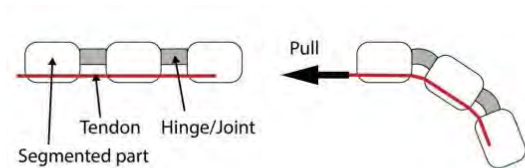
Рисунок 2 . Принцип роботи захвату з вбудованим кабелем. З відміченими сухожиллям, сегментом та з'єднанням
