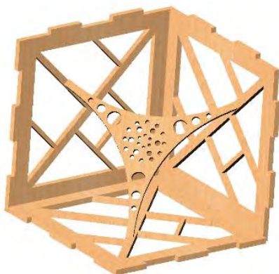
Рисунок 5. Модель каркасу. Частина кріплення електроніки
