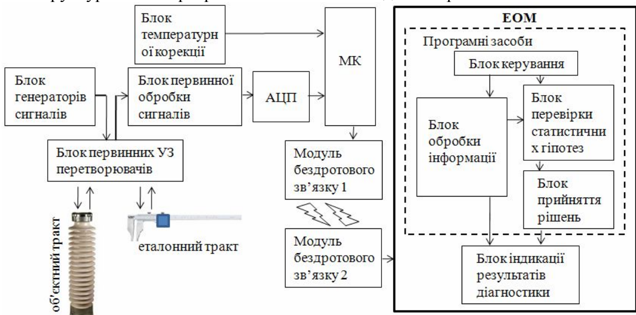
Рис. 2. Структурна схема системи діагностики технічного стану ПП.
